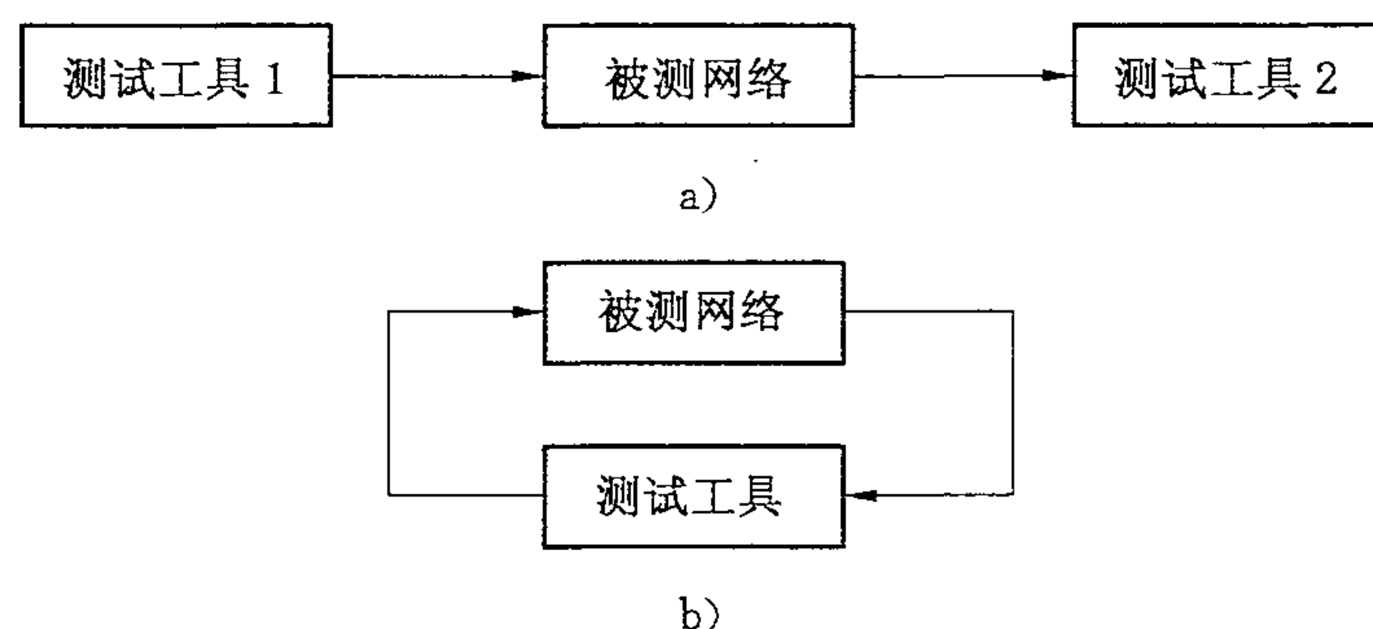
图 5 网络传输时延测试结构示意图
